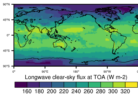
CERES-EBAF (264.2)
