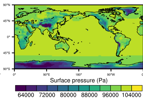
ERA5 (98572.1)
