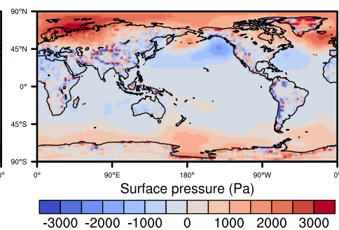
SCREAM minus ERA5 (-3.3)
