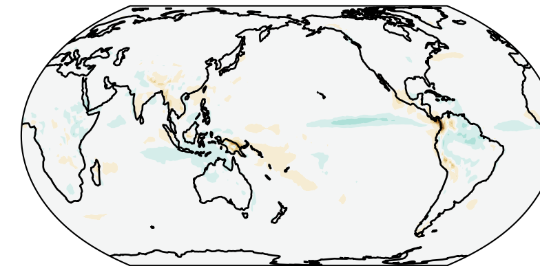
EAMv3 - EAMv2 (ANN)
