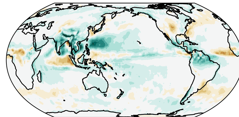
EAMv3 - GPCP (JJA) (Bias: 0.25 mm d -1 / RMSE: 1.17 mm d -1 / r : 0.91)
