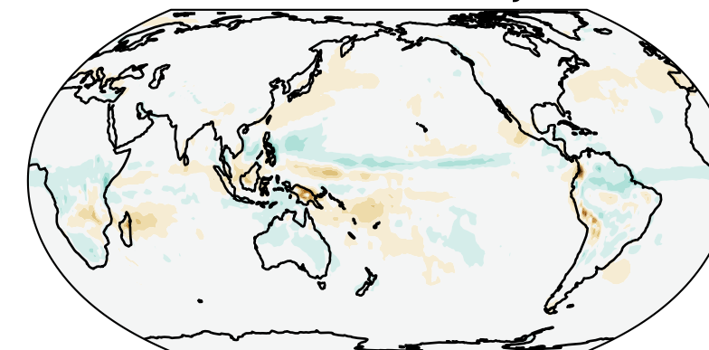
EAMv3 - EAMv2 (DJF)
