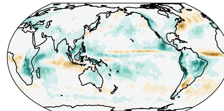
EAMv2 - GPCP (DJF) (Bias: 0.21 mm d -1 / RMSE: 1.18 mm d -1 / r : 0.90)
