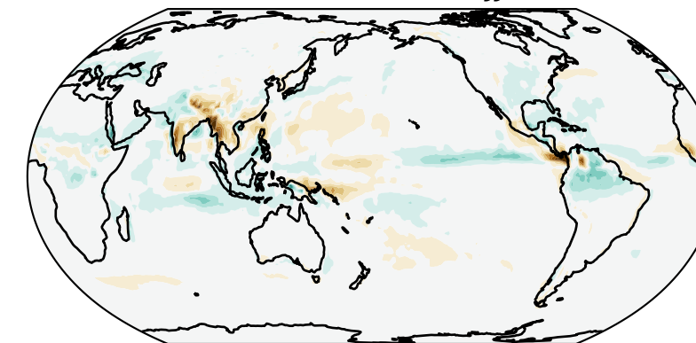
EAMv3 - EAMv2 (JJA)
