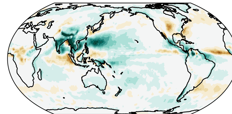
EAMv2 - GPCP (JJA) (Bias: 0.24 mm d -1 / RMSE: 1.33 mm d -1 / r : 0.89)
