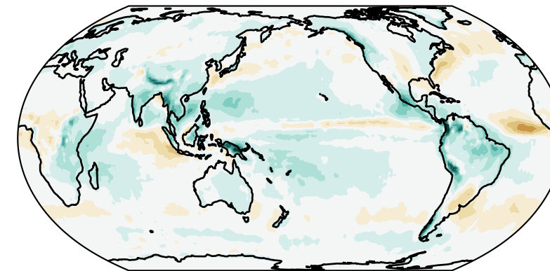
EAMv2 - GPCP (ANN) (Bias: 0.20 mm d -1 / RMSE: 0.90 mm d -1 / r : 0.91)
