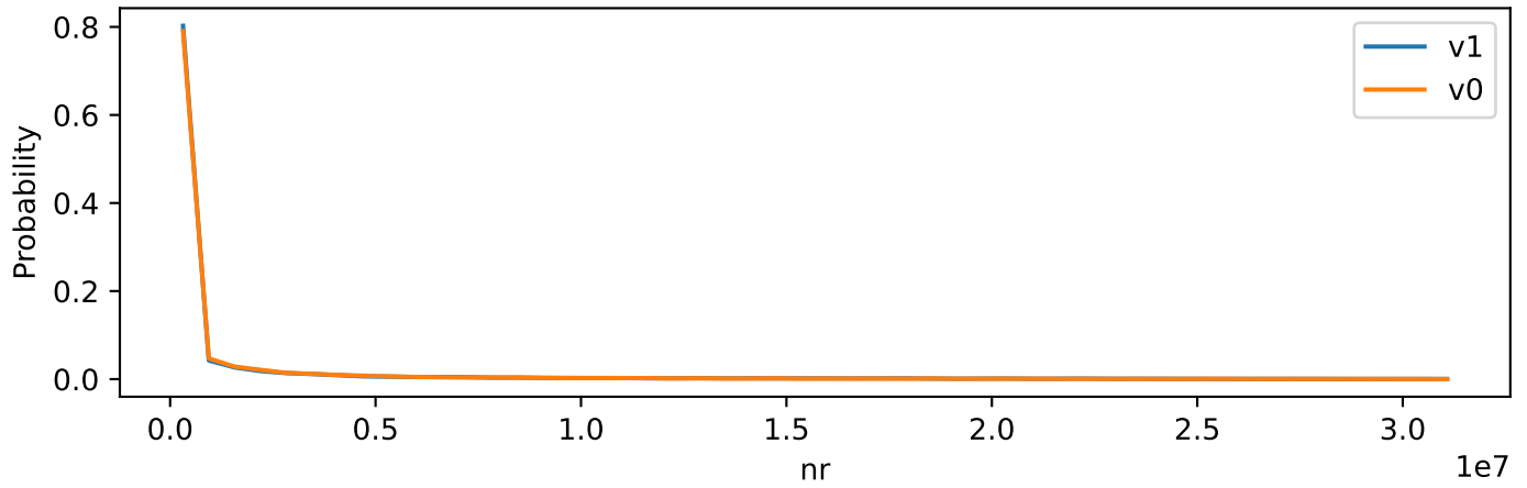
nr Global PDF, units=1/m2)
