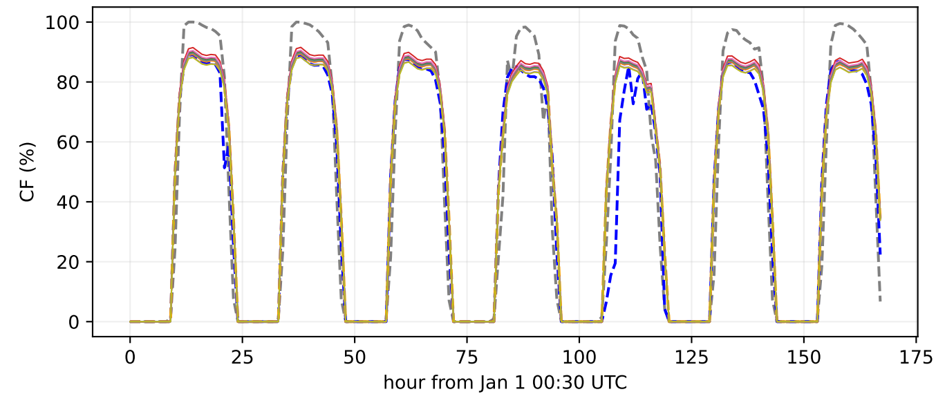
bus 806 | PMGD PFV PARQUE PVP ITIHUE
