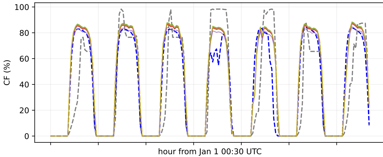
bus 805 | PMGD PFV PARQUE VALPARAISO
