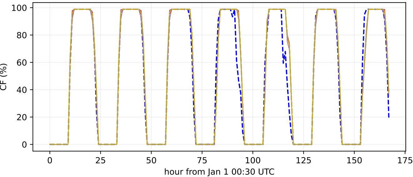
bus 1129 | PMGD PFV CUARZO
