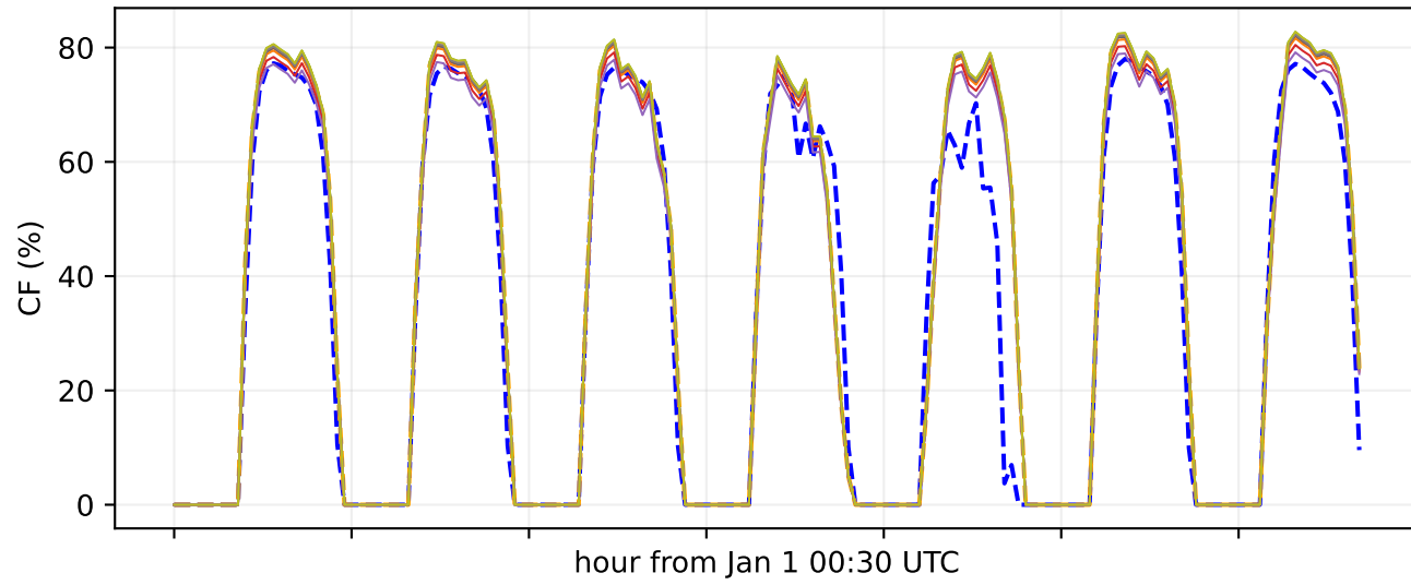
bus 1129 | PMGD PFV CUARZO
