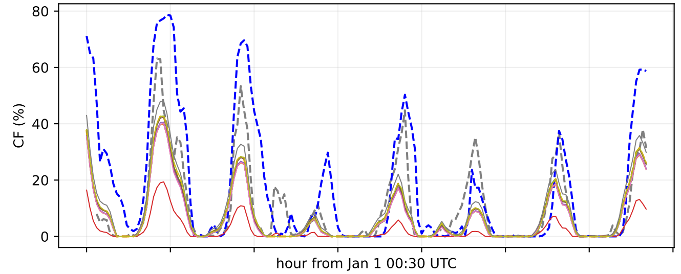
bus 317 | PE VALLE DE LOS VIENTOS
