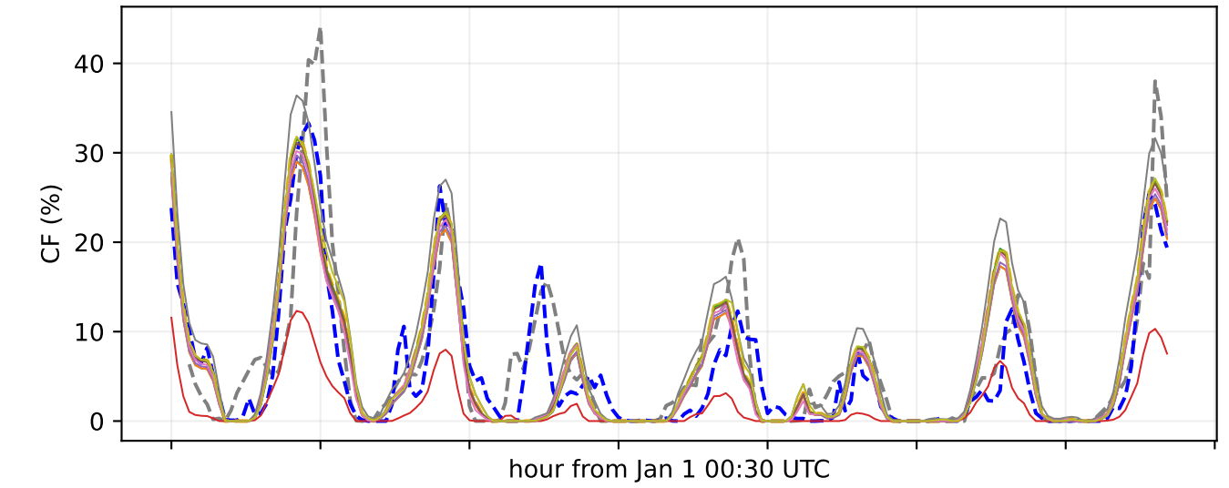
bus 563 | PE LA ESTRELLA
