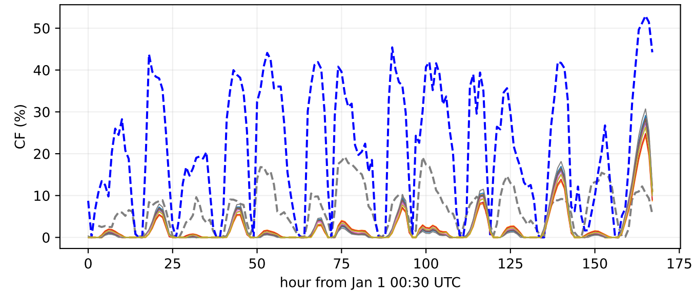
bus 1149 | PE HORIZONTE SUR
