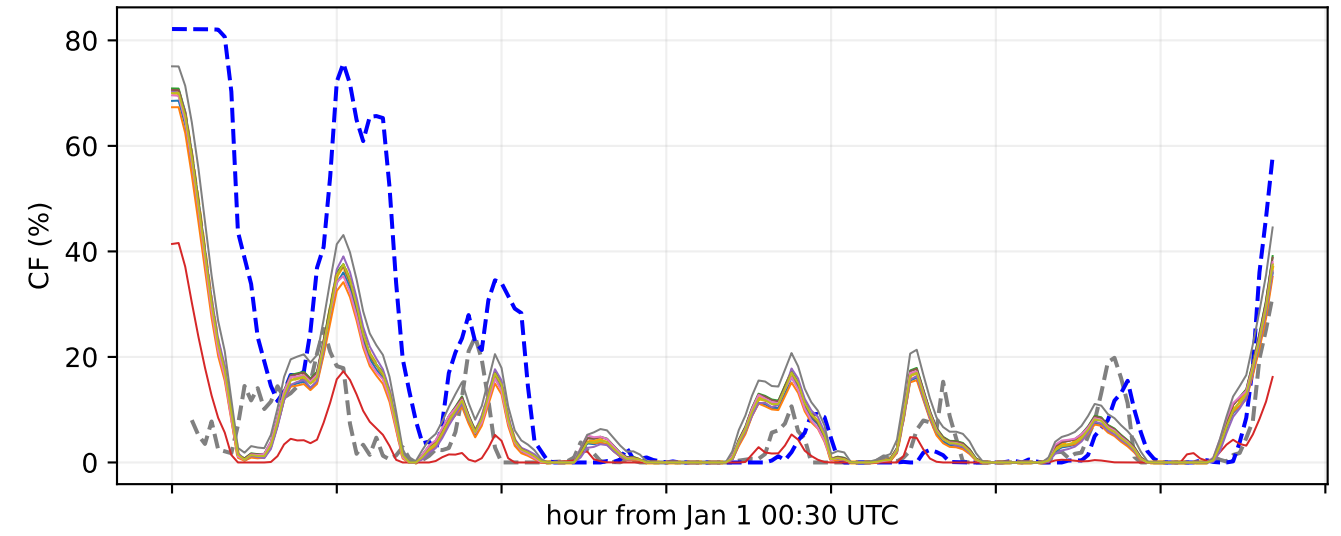
bus 262 | PE RENAICO I
