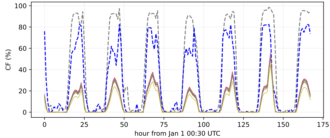
bus 317 | PE VALLE DE LOS VIENTOS
