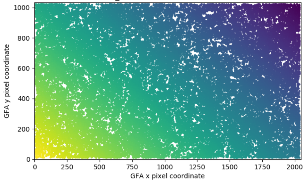
X_PTL ; 70647 stars ; GUIDE5
