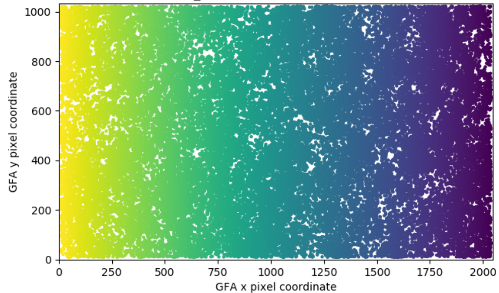
Y_PTL ; 69530 stars ; GUIDE7
