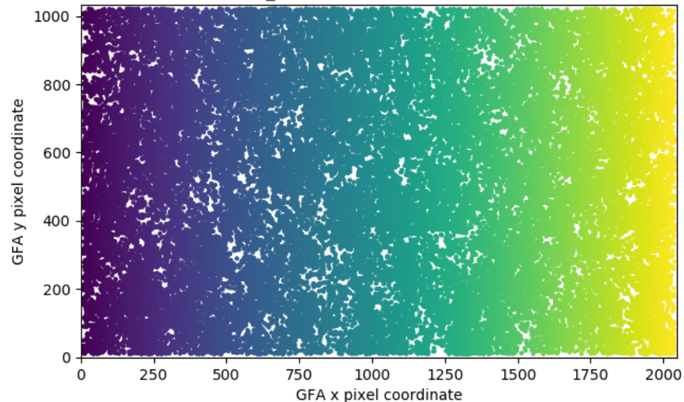
Y_PTL ; 67069 stars ; GUIDE2
