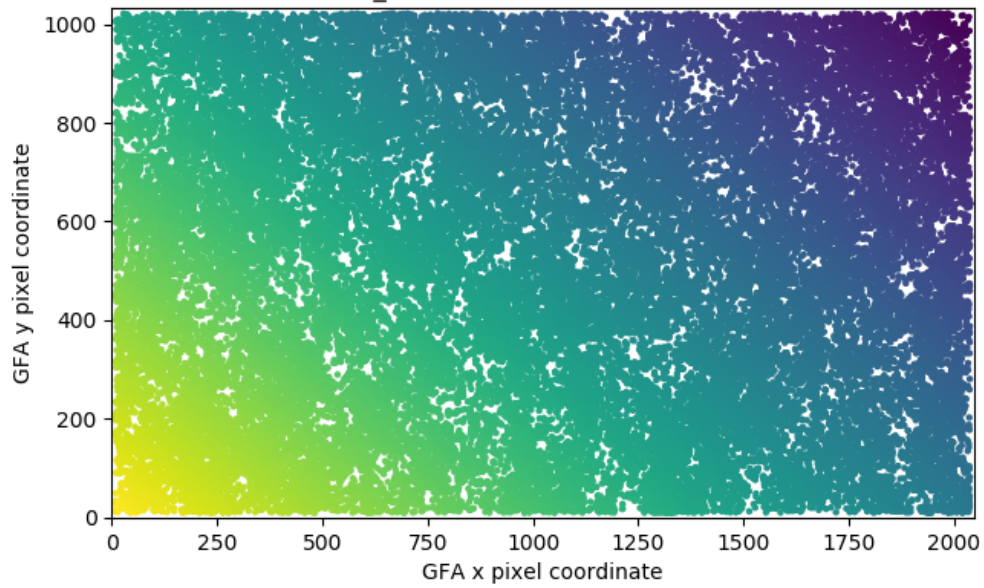
X_PTL ; 67069 stars ; GUIDE2
