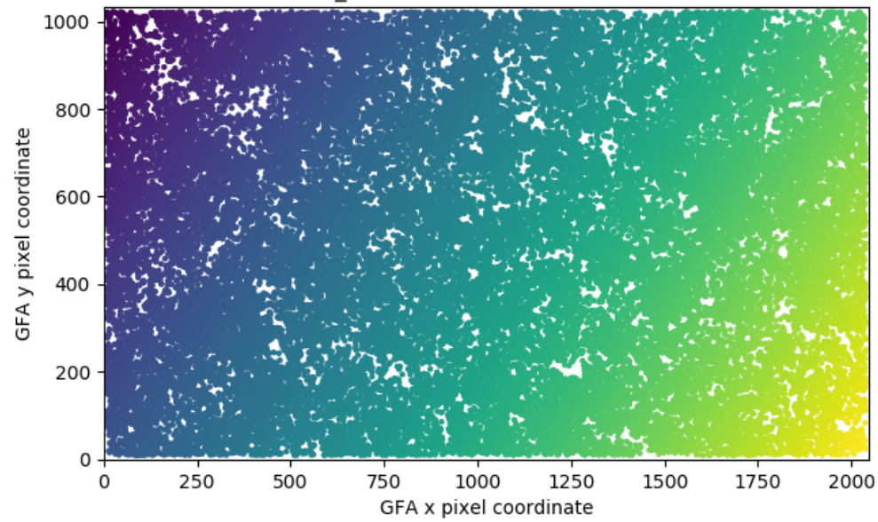
Y_PTL ; 64604 stars ; GUIDE0
