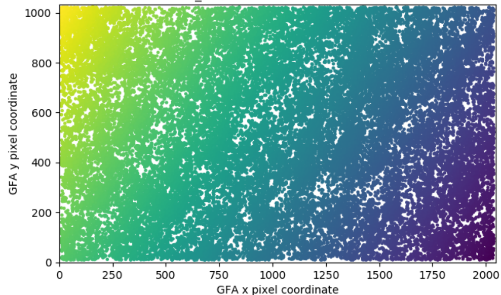
Y_PTL ; 55413 stars ; GUIDE8
