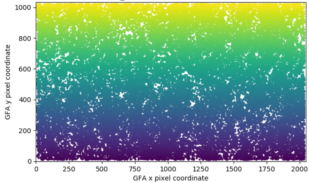
X_PTL ; 69530 stars ; GUIDE7
