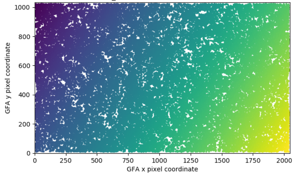
Y_PTL ; 70647 stars ; GUIDE5
