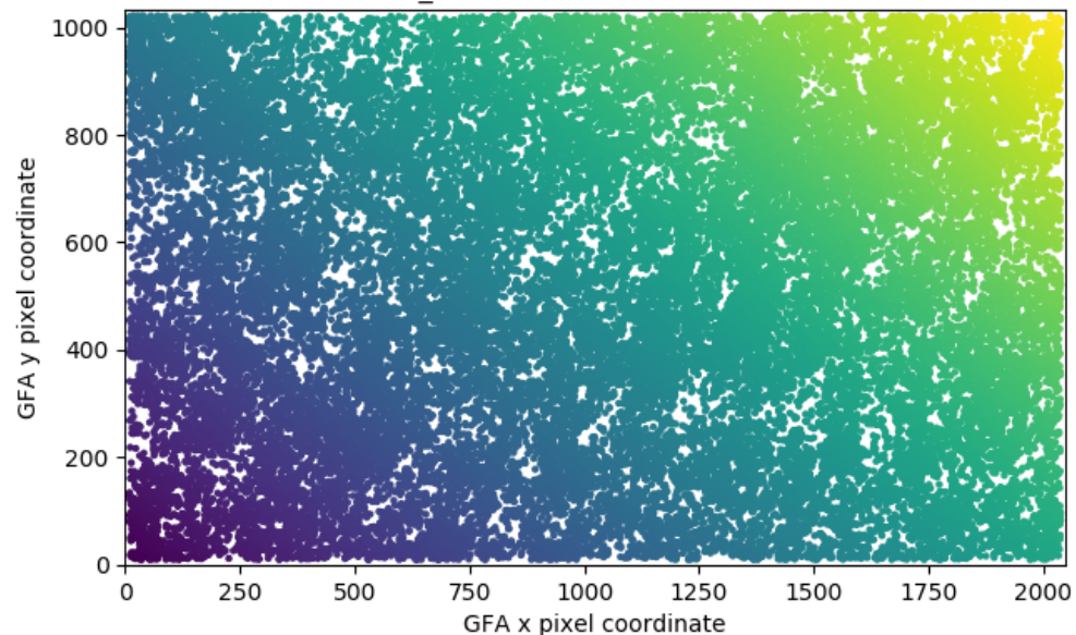
X_PTL ; 55413 stars ; GUIDE8
