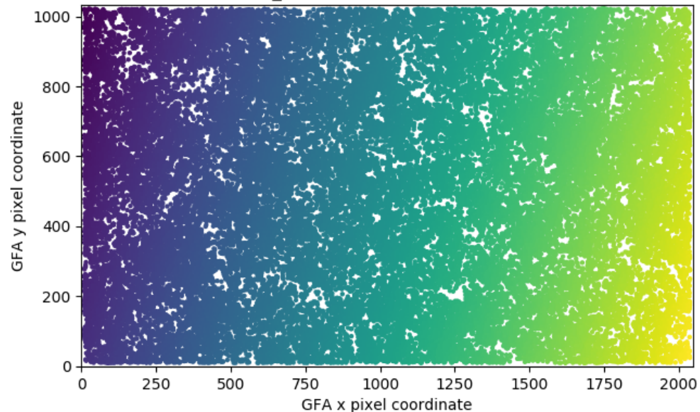
X_PTL ; 64604 stars ; GUIDE0
