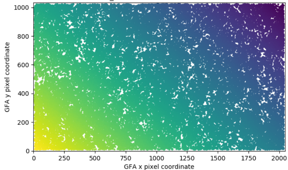
X_PTL ; 71161 stars ; GUIDE3
