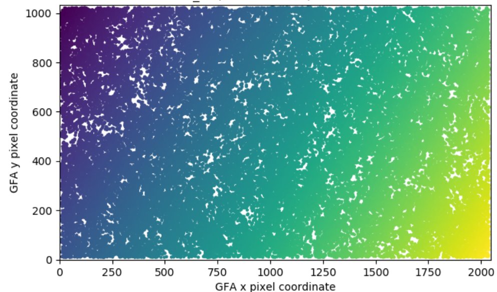
Y_PTL ; 71161 stars ; GUIDE3
