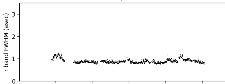
DESI GFA ; 20210707
