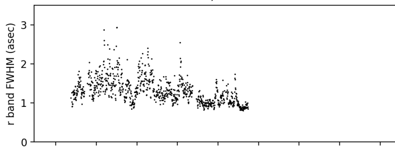
DESI GFA ; 20210704
