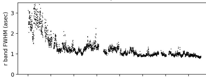
DESI GFA ; 20210708
