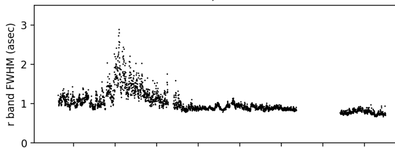
DESI GFA ; 20210706
