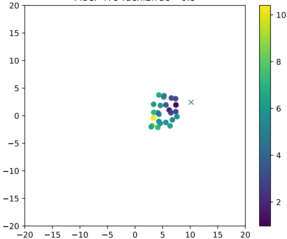
Fiber 4794dchi2frac= 0.9
