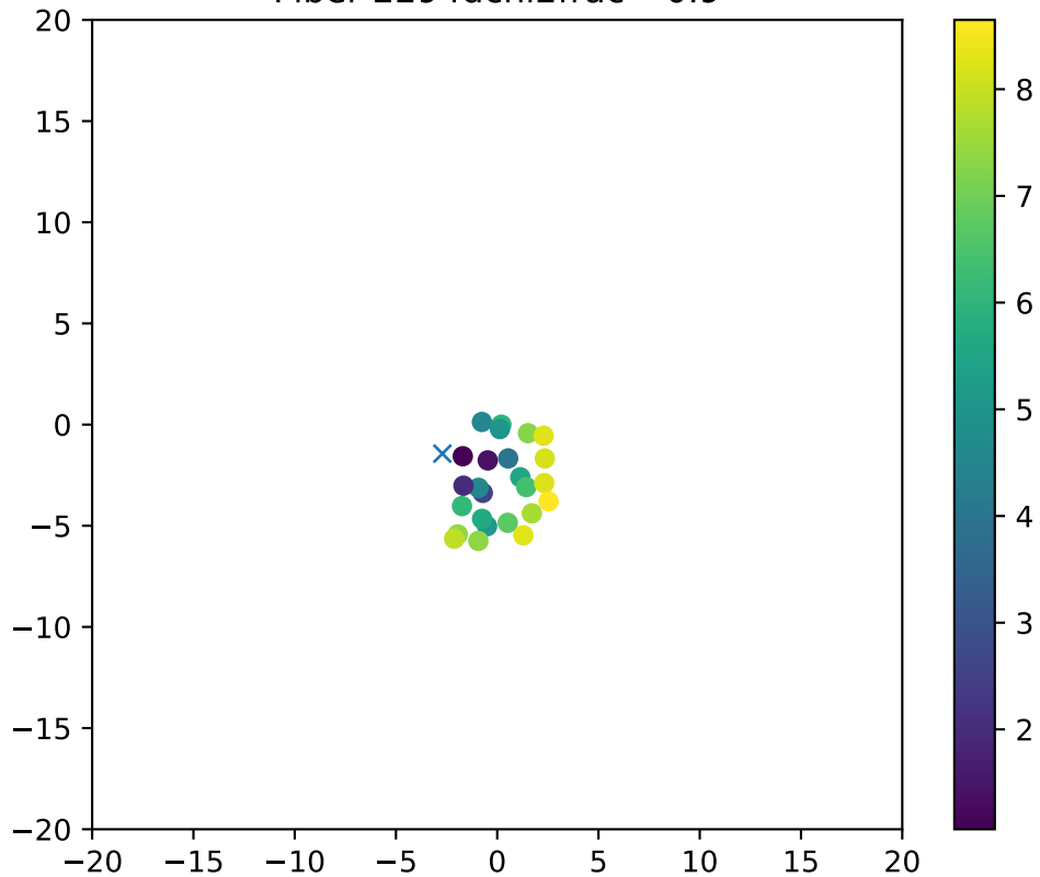
Fiber 2294dchi2frac= 0.9
