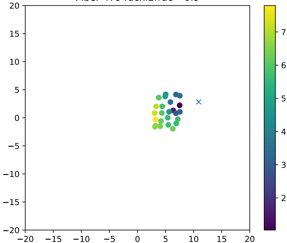
Fiber 4794dchi2frac= 0.9
