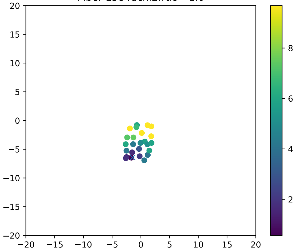
Fiber 1584dchi2frac= 1.0
