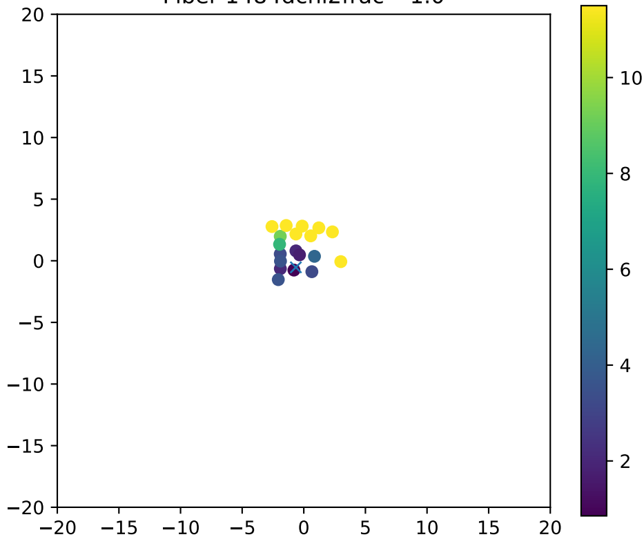
Fiber 1484dchi2frac= 1.0
