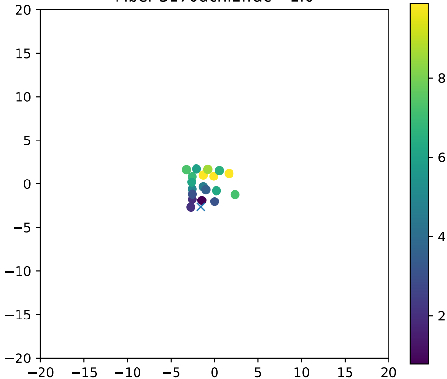
Fiber 3170dchi2frac= 1.0
