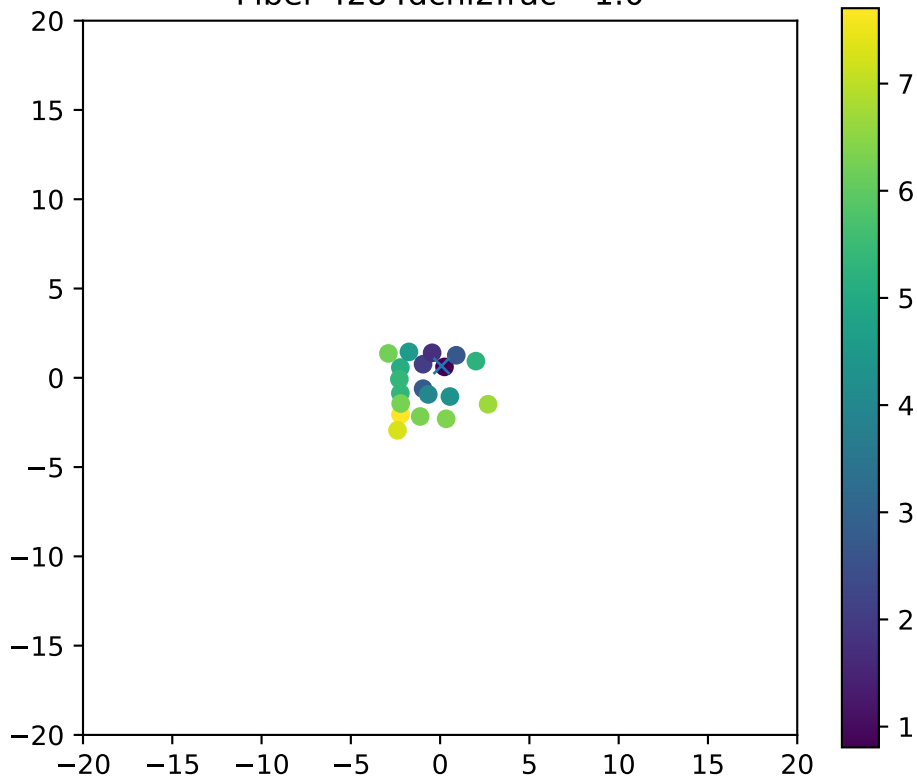
Fiber 4284dchi2frac= 1.0
