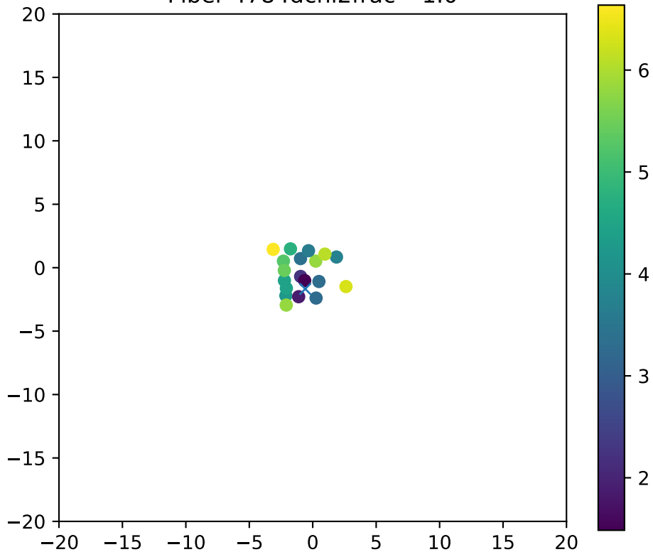
Fiber 4784dchi2frac= 1.0
