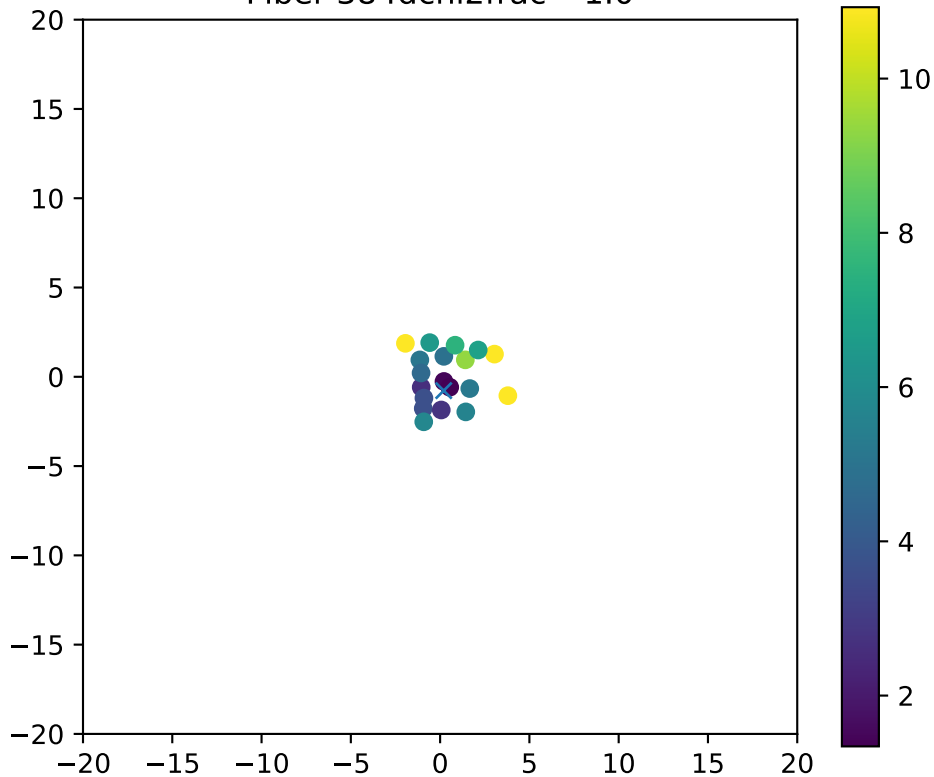
Fiber 384dchi2frac= 1.0
