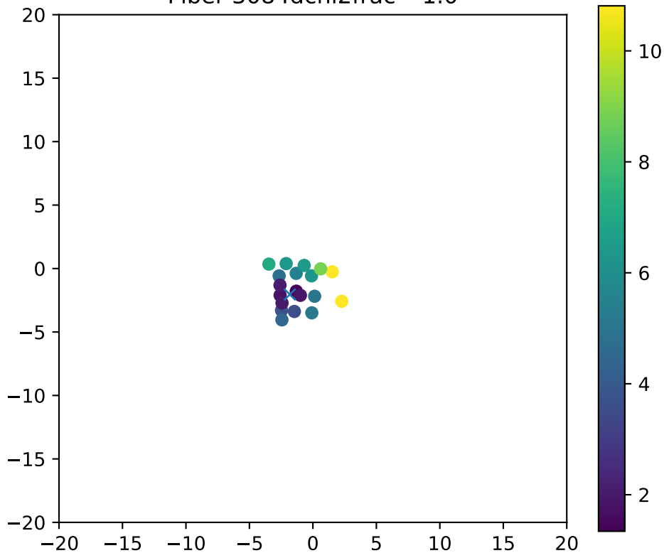
Fiber 3084dchi2frac= 1.0
