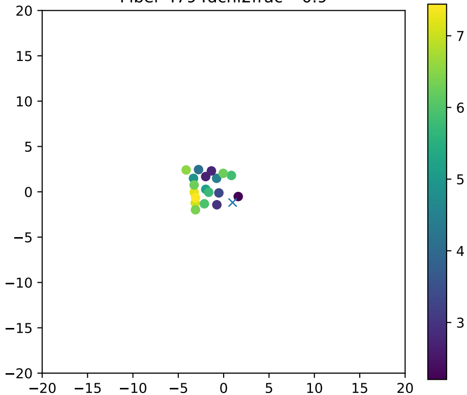
Fiber 4794dchi2frac= 0.9
