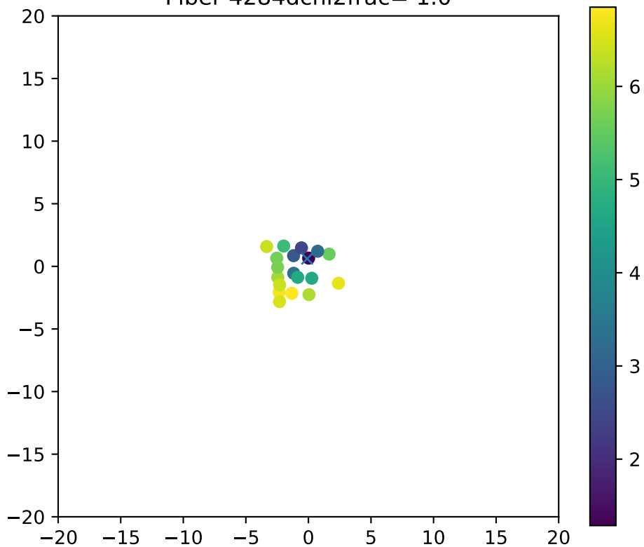
Fiber 4284dchi2frac= 1.0
