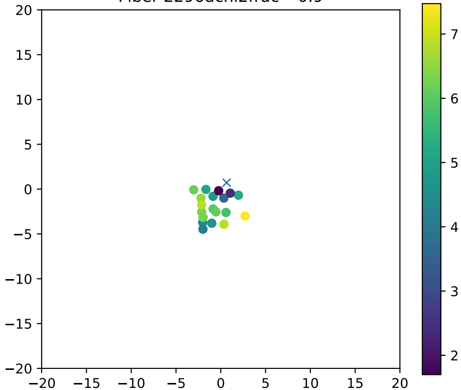
Fiber 2296dchi2frac= 0.9
