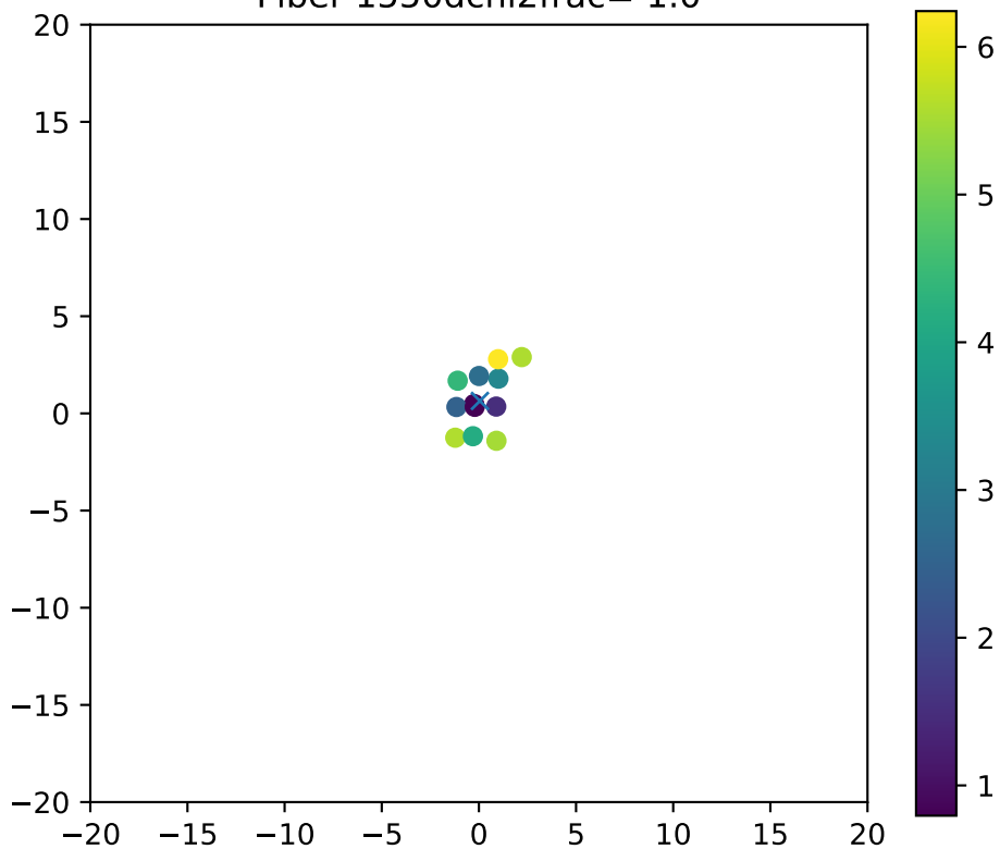
Fiber 1550dchi2frac= 1.0
