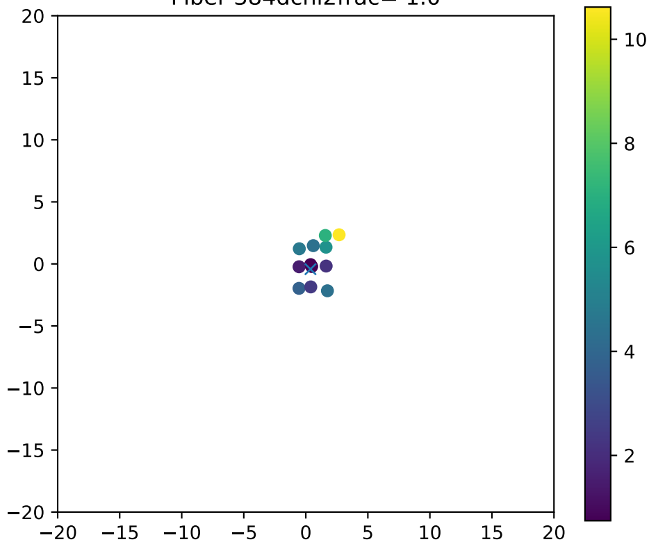
Fiber 384dchi2frac= 1.0
