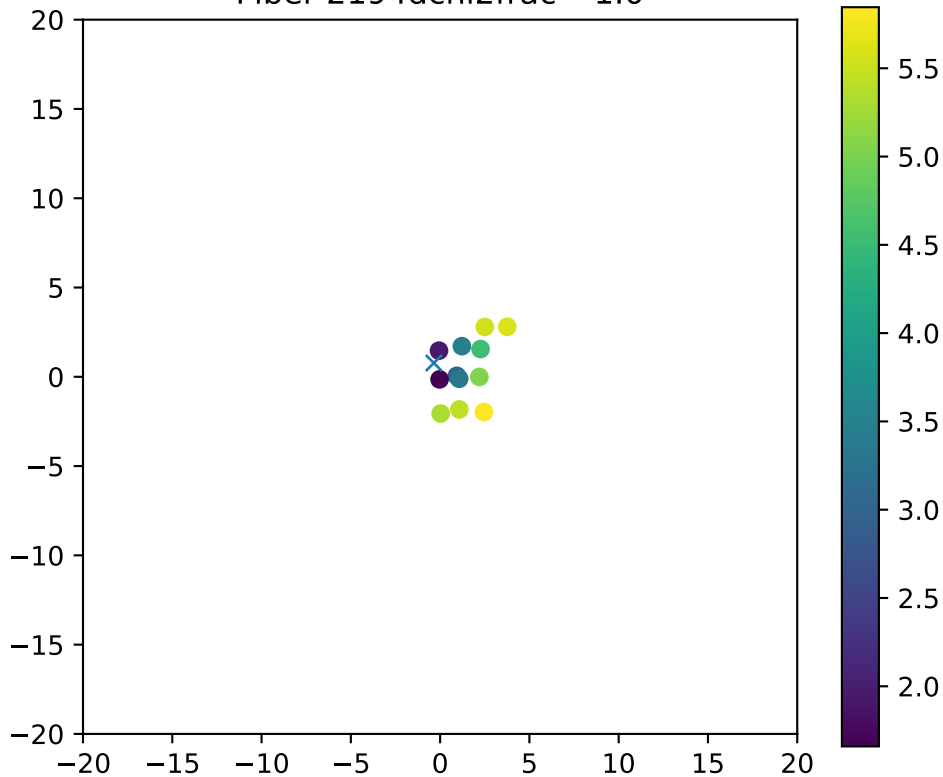
Fiber 2194dchi2frac= 1.0
