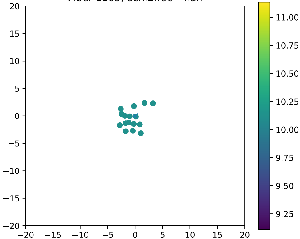
Fiber 1163, dchi2frac= nan
