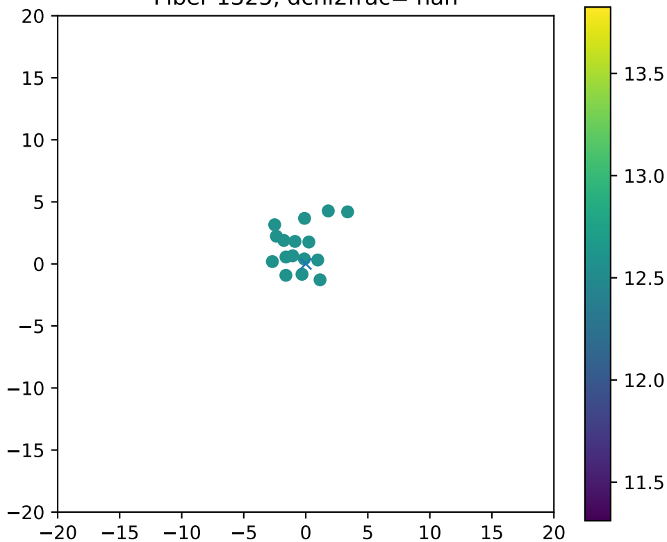
Fiber 1325, dchi2frac= nan
