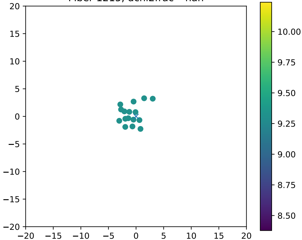
Fiber 1215, dchi2frac= nan
