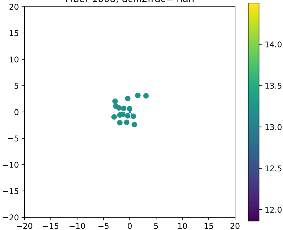
Fiber 1008, dchi2frac= nan
