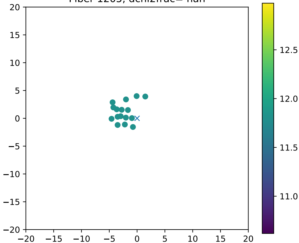
Fiber 1205, dchi2frac= nan
