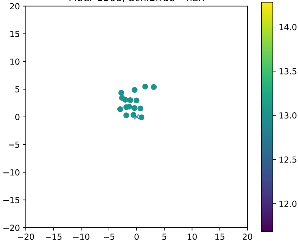
Fiber 1266, dchi2frac= nan
