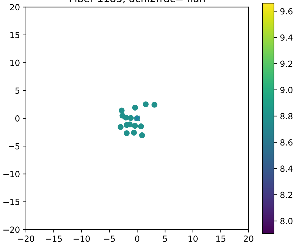
Fiber 1185, dchi2frac= nan
