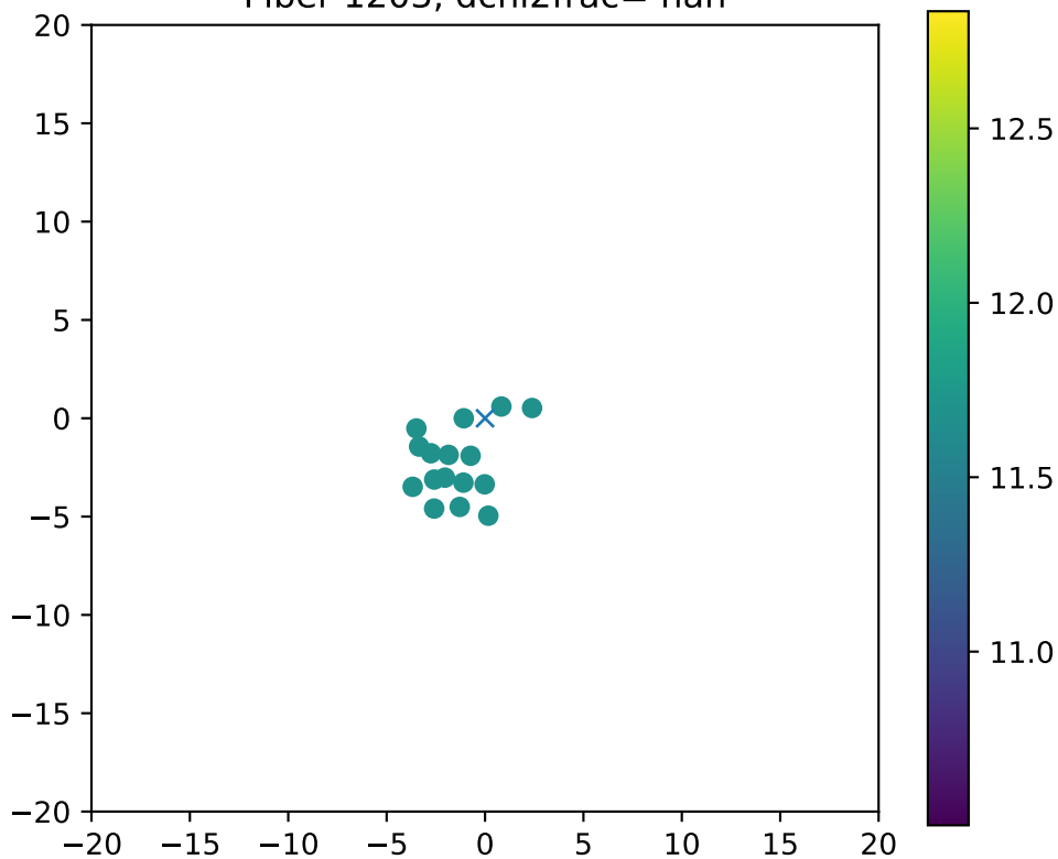
Fiber 1203, dchi2frac= nan
