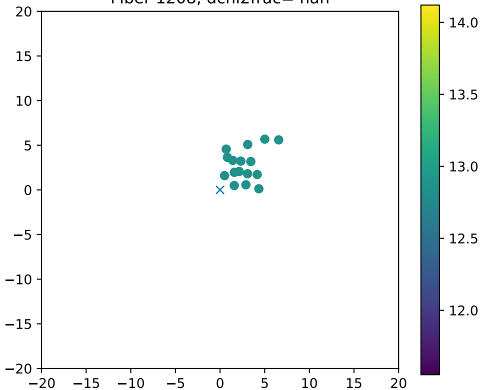
Fiber 1208, dchi2frac= nan
