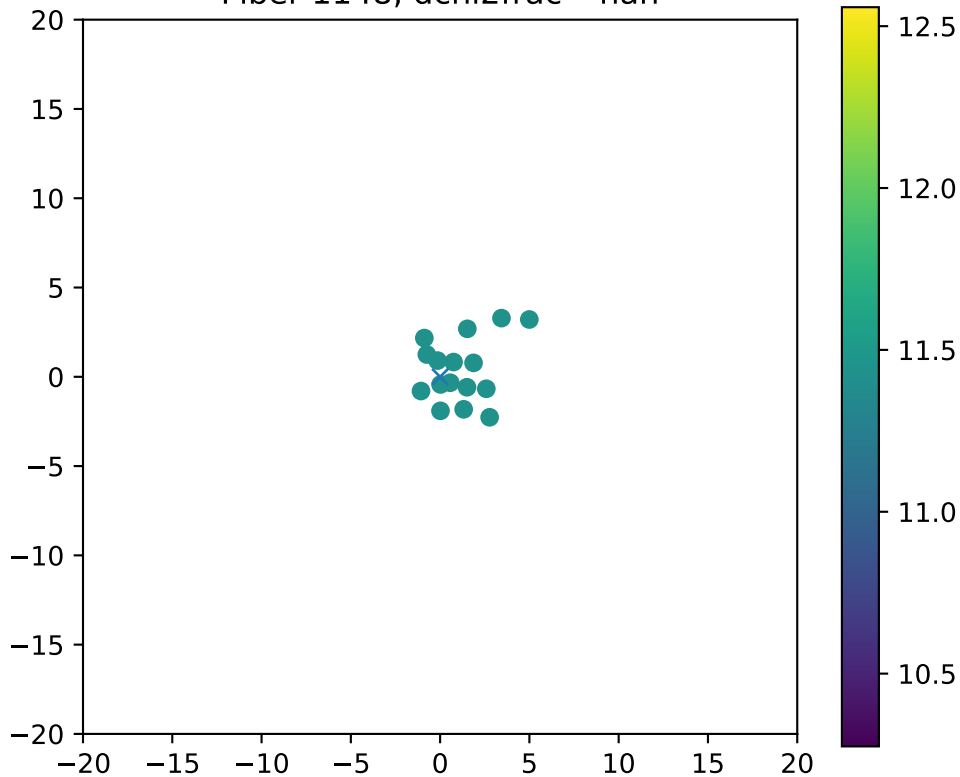
Fiber 1148, dchi2frac= nan
