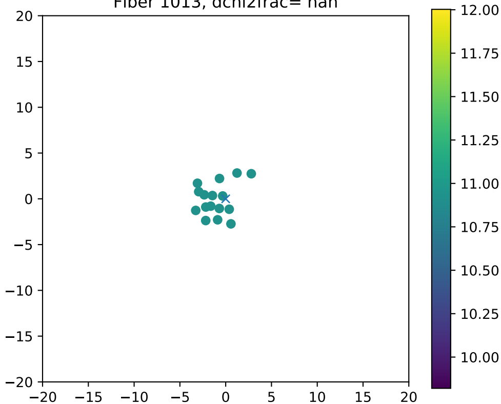
Fiber 1013, dchi2frac= nan
