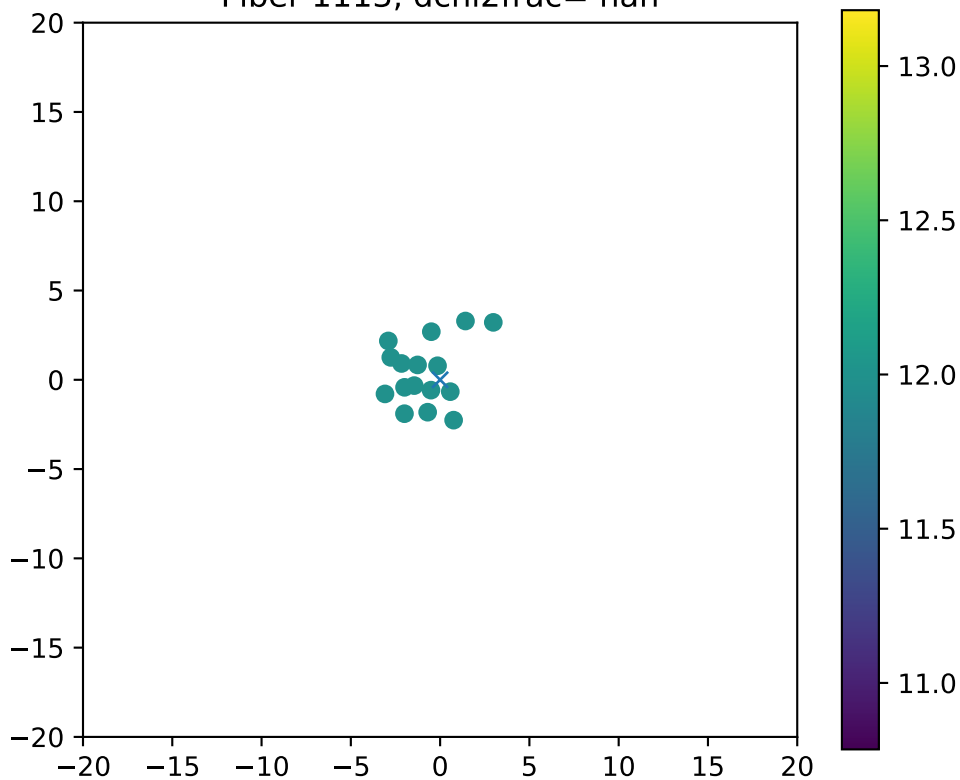
Fiber 1113, dchi2frac= nan
