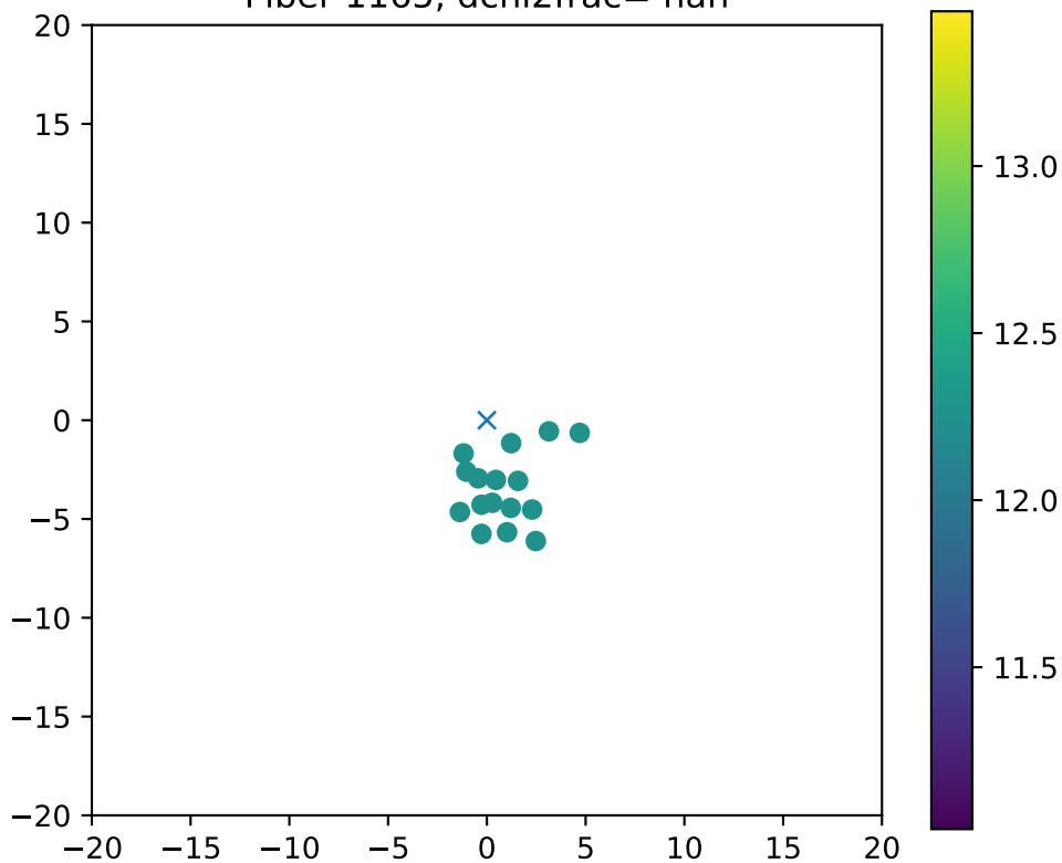
Fiber 1165, dchi2frac= nan
