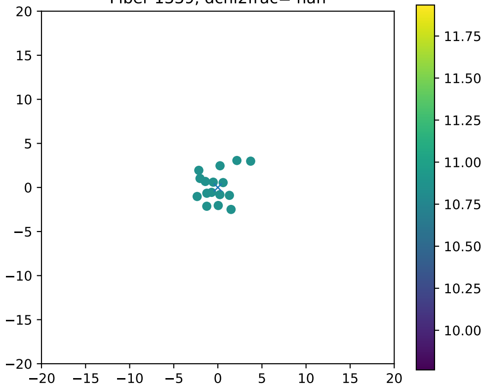
Fiber 1339, dchi2frac= nan
