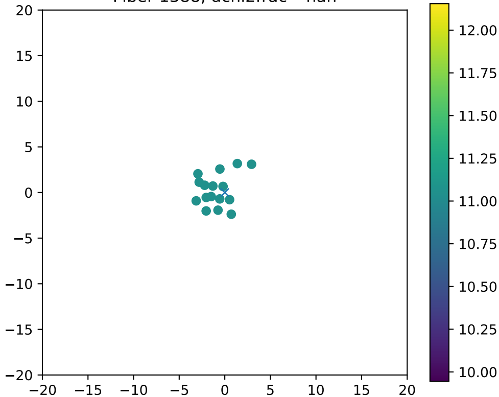
Fiber 1388, dchi2frac= nan
