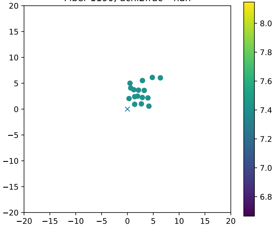
Fiber 1190, dchi2frac= nan
