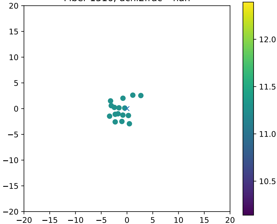
Fiber 1316, dchi2frac= nan
