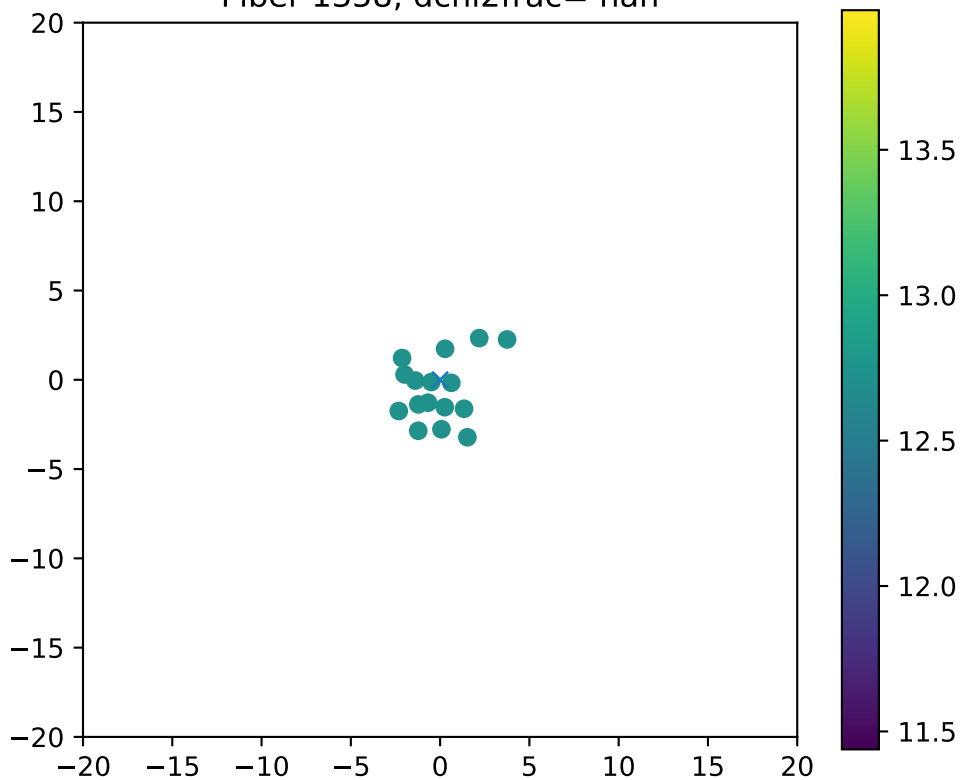
Fiber 1358, dchi2frac= nan
