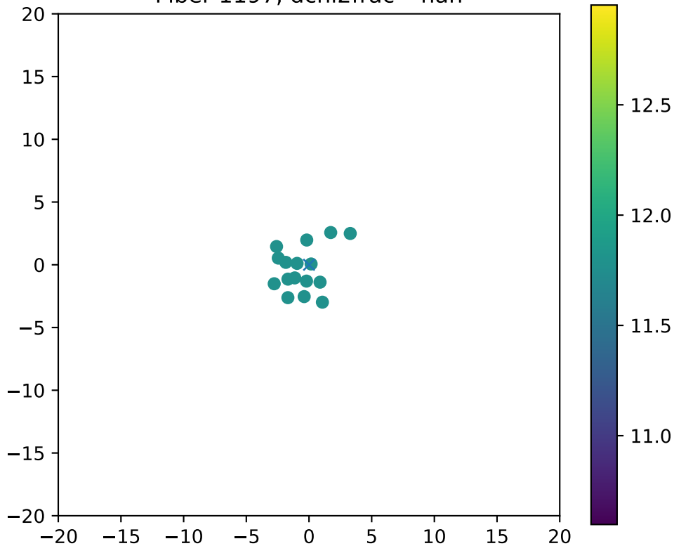
Fiber 1197, dchi2frac= nan
