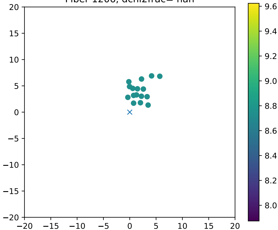
Fiber 1206, dchi2frac= nan
