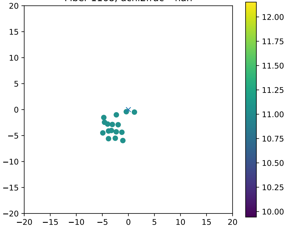
Fiber 1168, dchi2frac= nan
