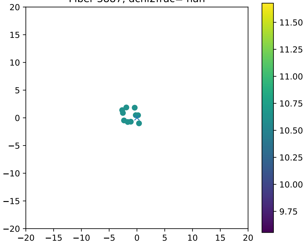
Fiber 3887, dchi2frac= nan
