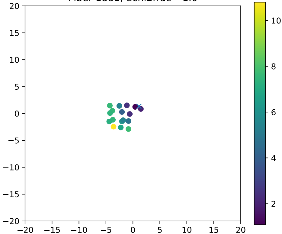
Fiber 1881, dchi2frac= 1.0
