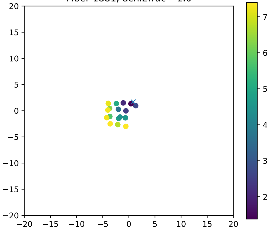
Fiber 1881, dchi2frac= 1.0
