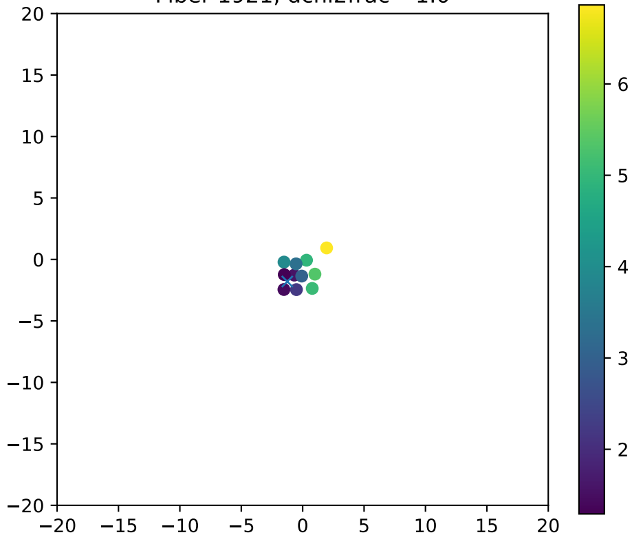
Fiber 1921, dchi2frac= 1.0
