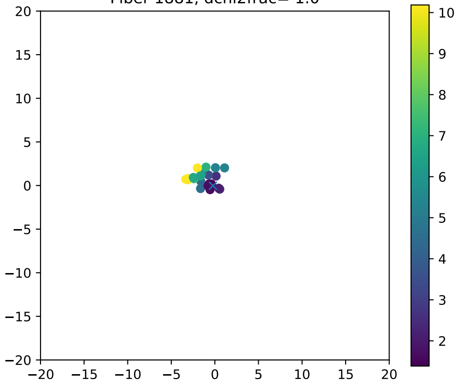
Fiber 1881, dchi2frac= 1.0
