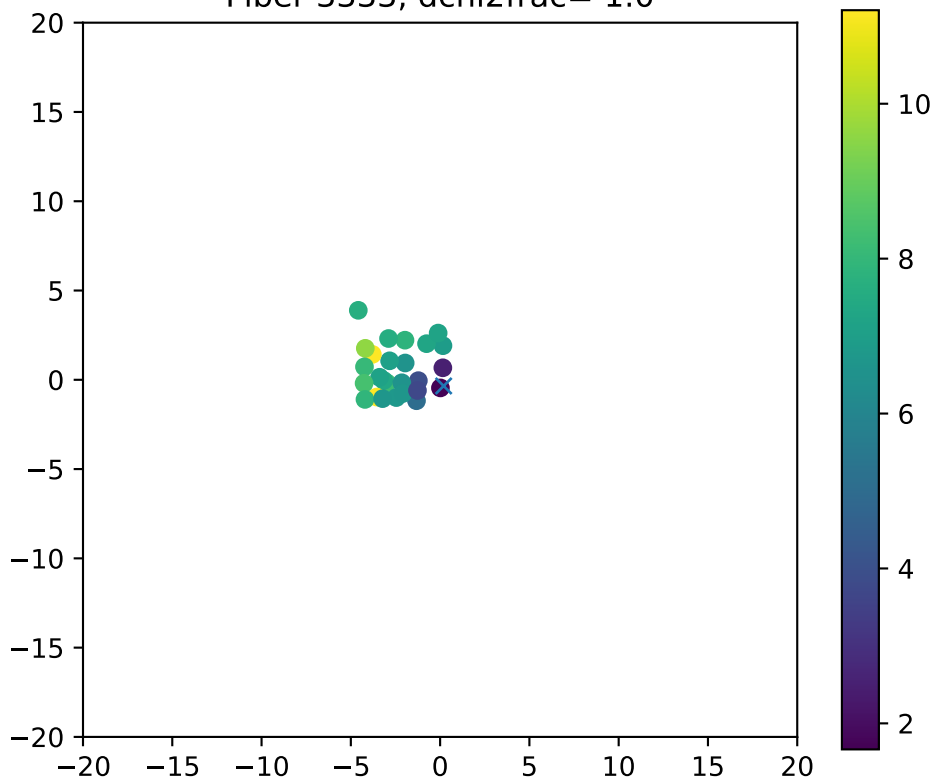
Fiber 3333, dchi2frac= 1.0
