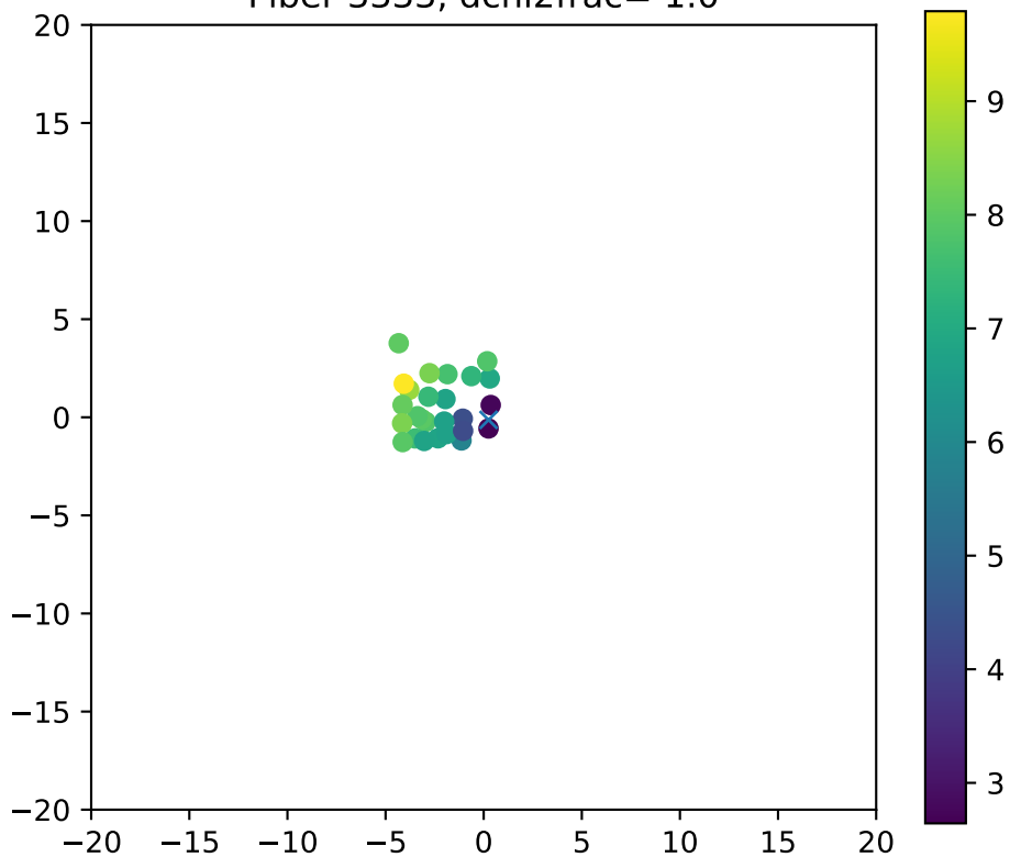
Fiber 3333, dchi2frac= 1.0
