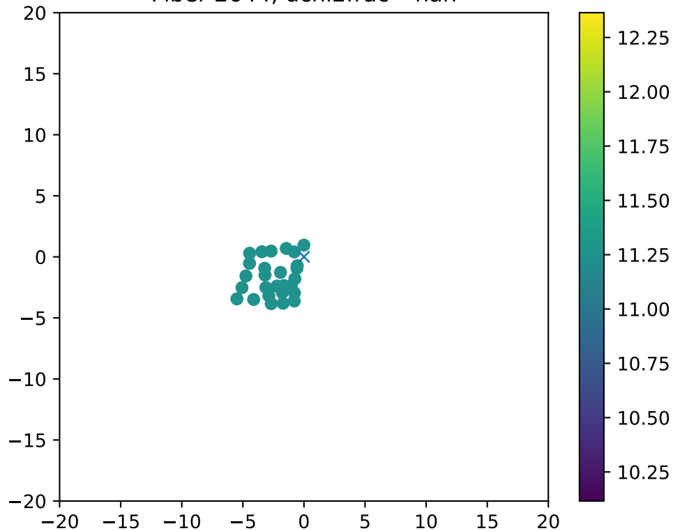
Fiber 2644, dchi2frac= nan
