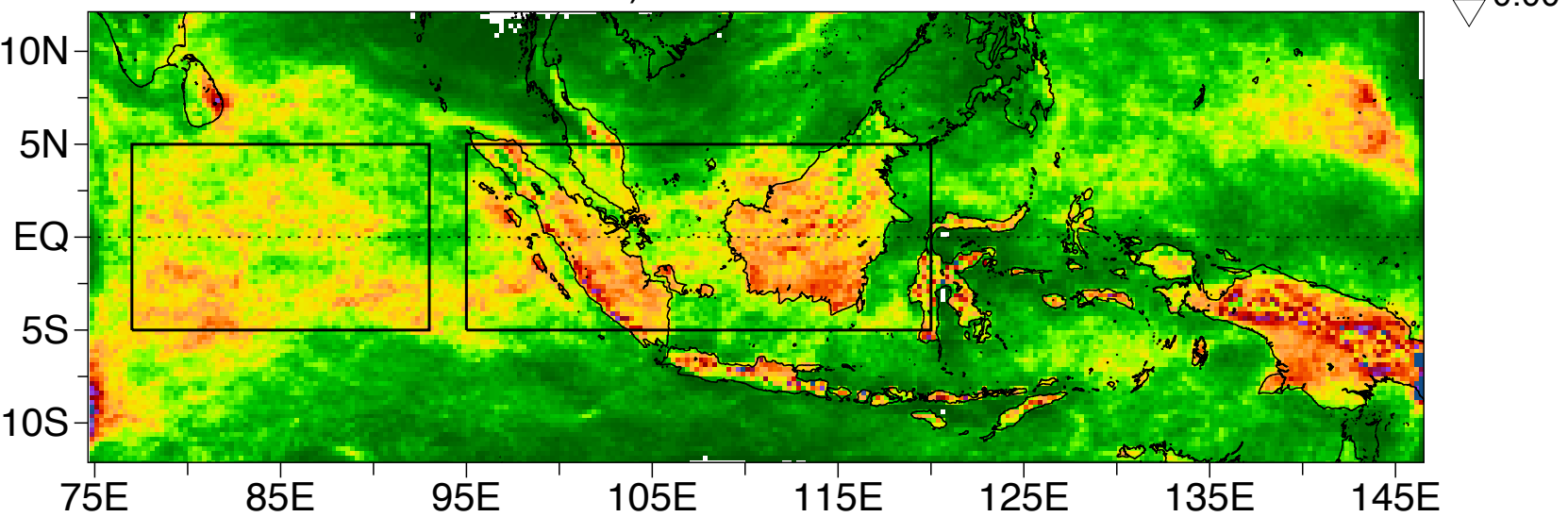
c) WRF NODIURC
