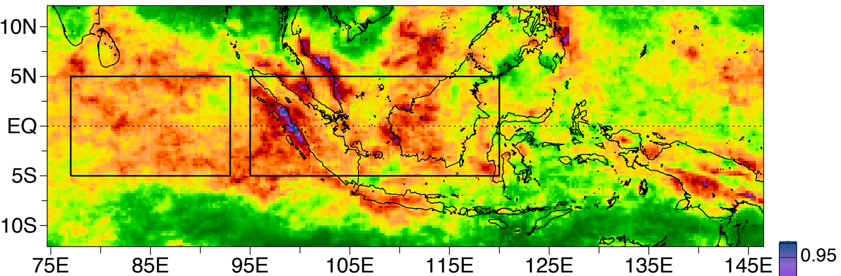
b) WRF CONTROL
