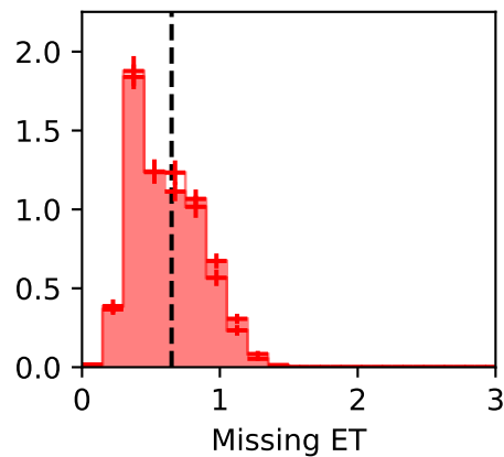
MET
