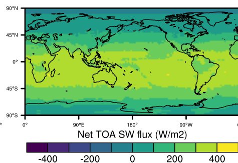
CERES-EBAF (247.7)
