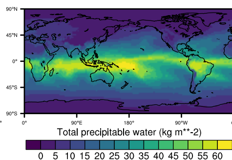
ERA5 (24.3)
