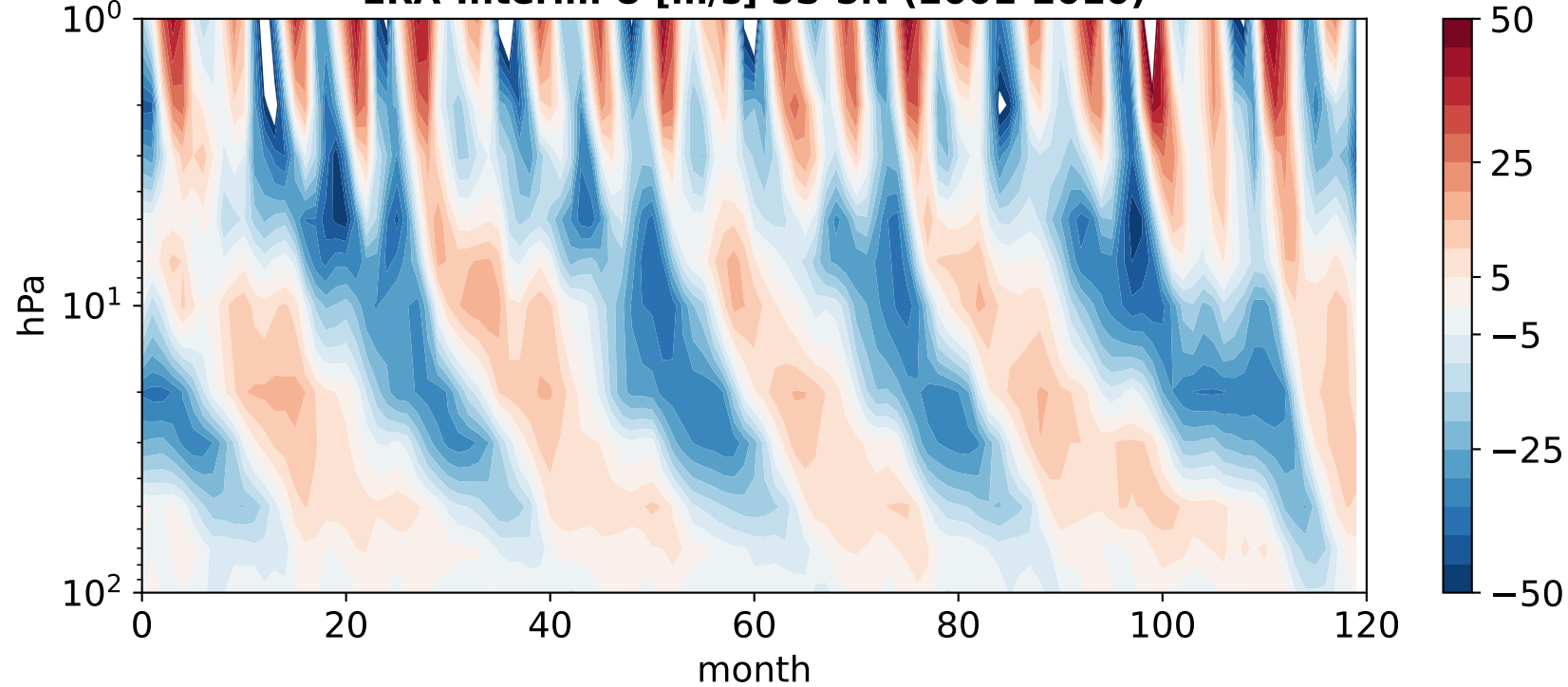
ERA-Interim U [m/s] 5S-5N (2001-2010)
