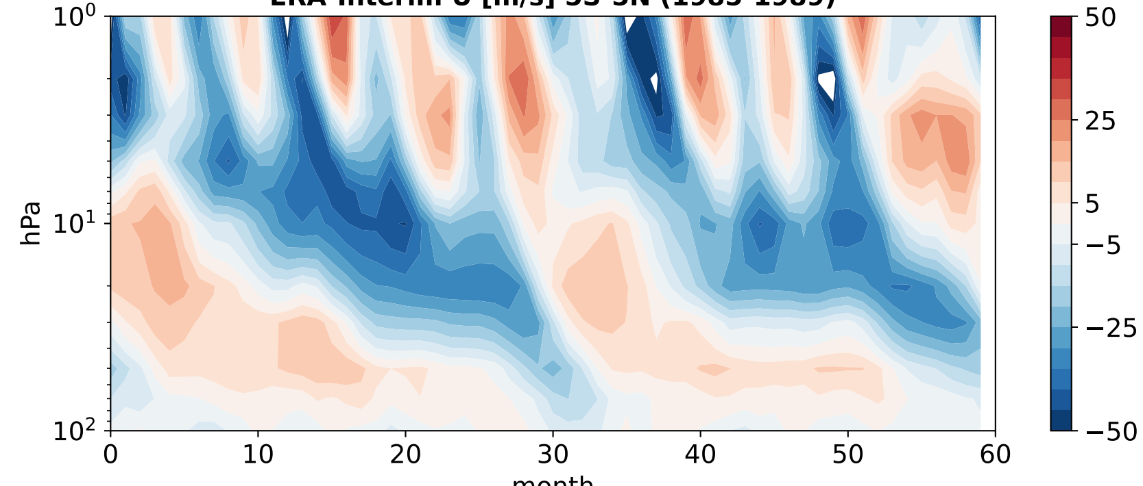
ERA-Interim U [m/s] 5S-5N (1985-1989)
