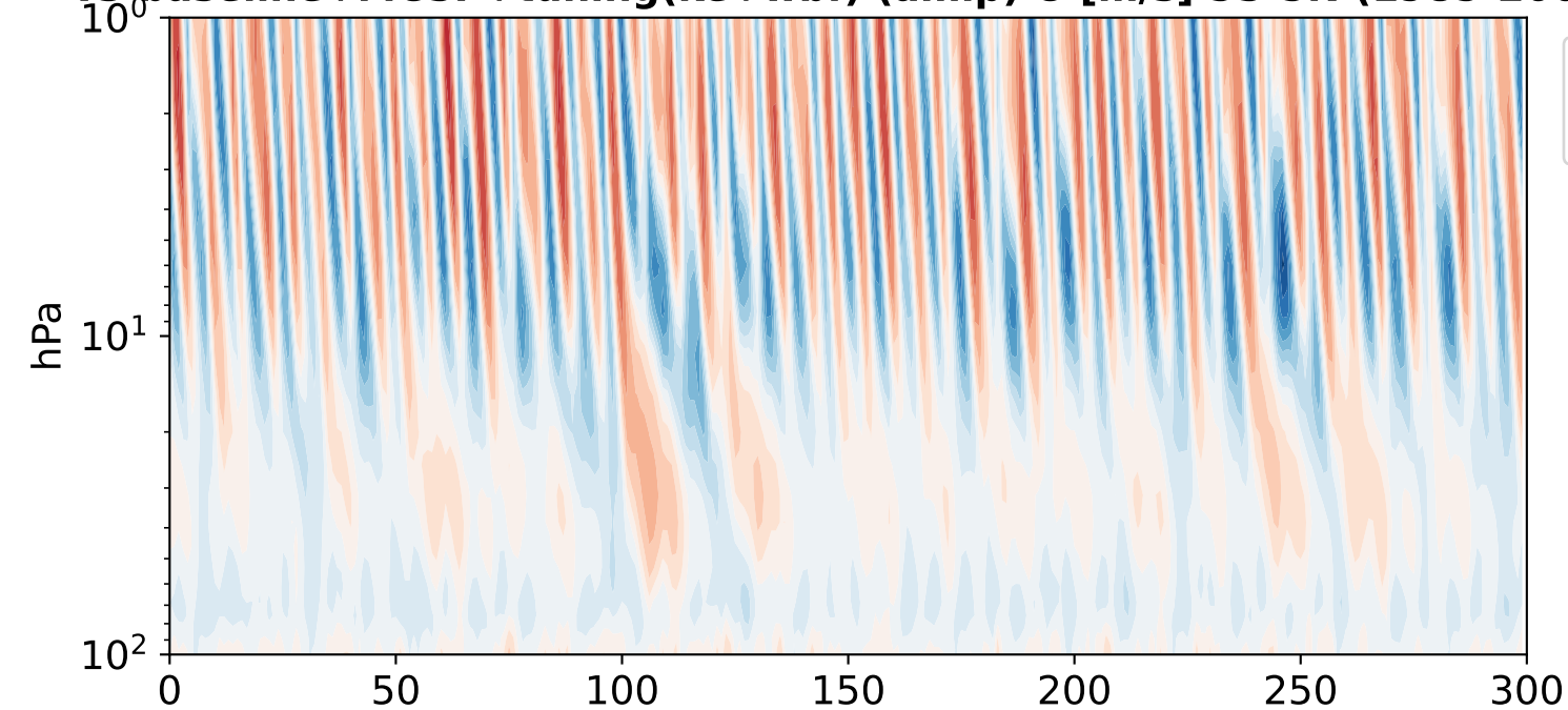
v3 baseline+MCSP+tuning(ke+wbf) (amip) U [m/s] 5S-5N (1985-2009)
