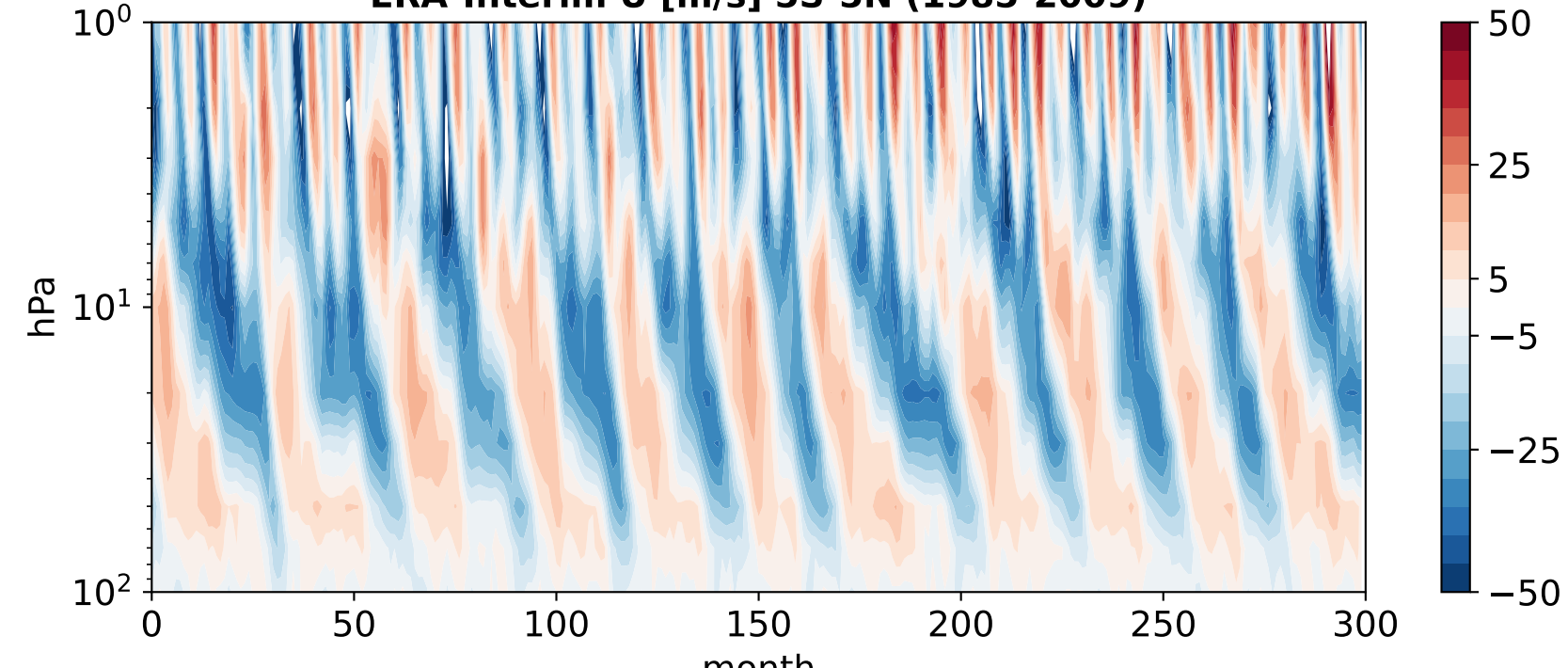
ERA-Interim U [m/s] 5S-5N (1985-2009)
