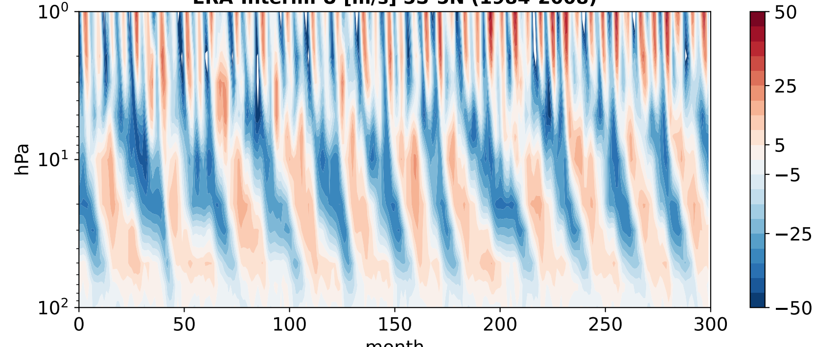
ERA-Interim U [m/s] 5S-5N (1984-2008)
