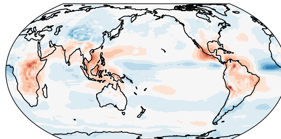
EAMv3 - CERES-EBAF (Bias: -1.01 \text{ W m}^{-2} / RMSE: 4.21 \text{ W m}^{-2} / r : 0.94)
