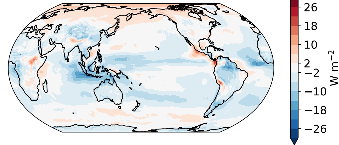
EAMv2 - CERES-EBAF (Bias: -2.08 \text{ W m}^{-2} / RMSE: 4.80 \text{ W m}^{-2} / r : 0.92)
