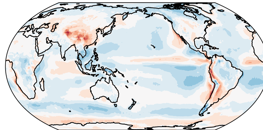
EAMv3 - CERES-EBAF (Bias: -3.88 \text{ W m}^{-2} / RMSE: 9.95 \text{ W m}^{-2} / r : 0.90)
