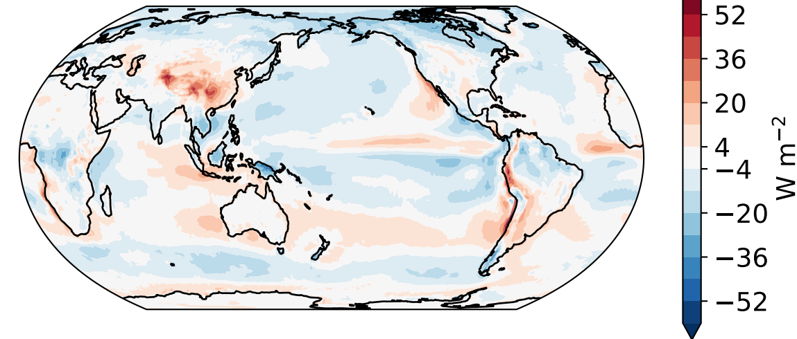
EAMv2 - CERES-EBAF (Bias: -2.54 \text{ W m}^{-2} / RMSE: 9.21 \text{ W m}^{-2} / r : 0.91)
