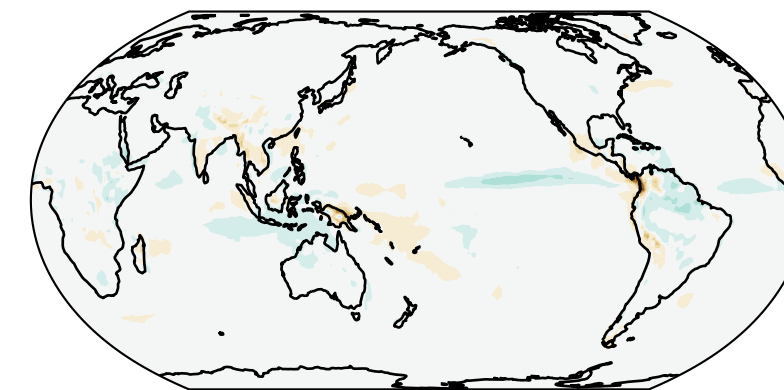
Precipitation rate (ANN) EAMv3 - EAMv2
