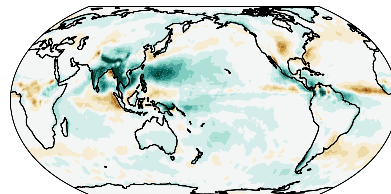
Precipitation rate (JJA) EAMv2 - GPCP
