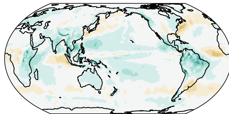
Precipitation rate (ANN) EAMv3 - GPCP
