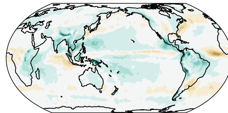
Precipitation rate (ANN) EAMv2 - GPCP
