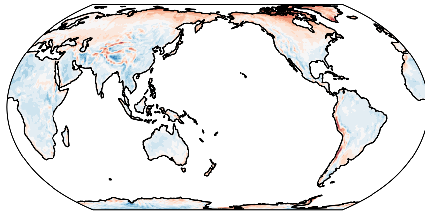
2-m Air Temperature: EAMv2 - ERA5 (Bias: -0.21 K / RMSE: 2.19 K/ r : 0.99)
