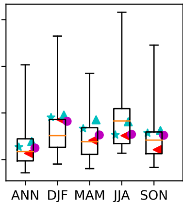
(g) u-200 ( \text{m s}^{-1} )
