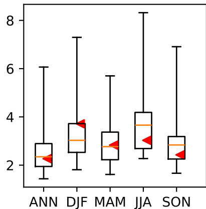
(g) u-200 ( \text{m s}^{-1} )
