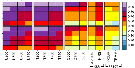
(d) Temporal correlation, mid-latitudes
