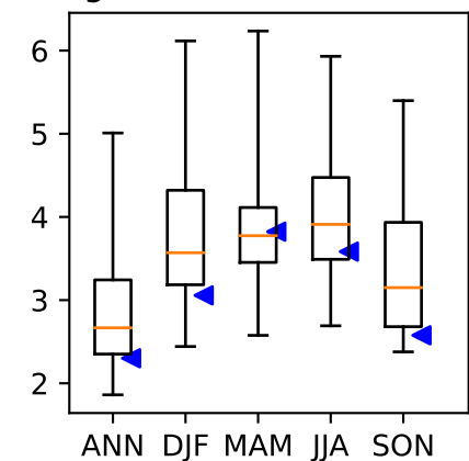
(g) u-200 ( \text{m s}^{-1} )
