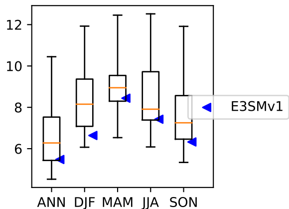
(f) SLP (hPa)
