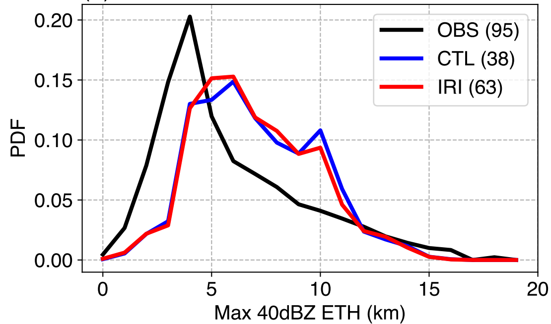
(d) MCS Max 40dBZ ETH
