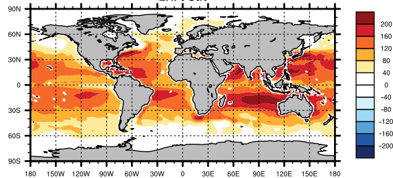
LHF: Ctrl
